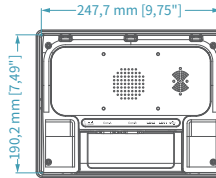
背視圖
