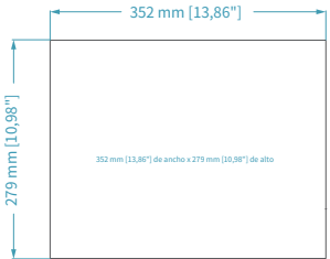
開孔尺寸
