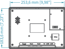
背視圖
