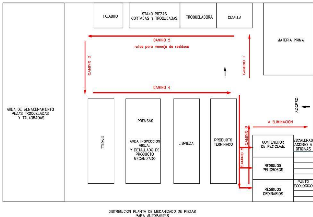
Figura 1 - Rutas de evacuación de los residuos planta Giravan SAS
